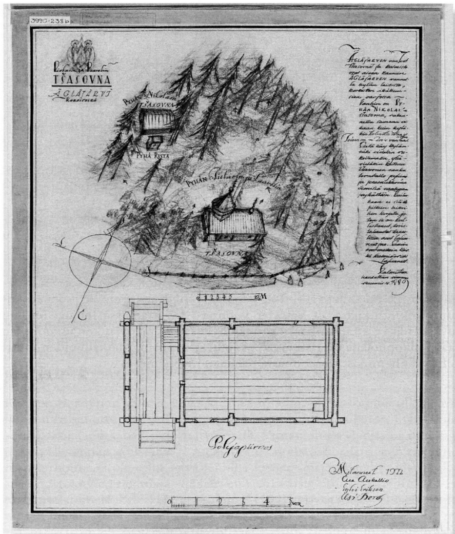
KUVA: Teknillinen Korkeakoulu teetti vuonna 1922 Ägläjärven kalmistoalueen ja nuoremman tsasounan mittapiirustukset, jotka ovat Elsa Arokallion, Elsi Borgin ja Sylvi Eriksonin piirtämiä. Piirroksessa kalmistoalueesta näkyy myös ristikatos, samoin tieto, että vanhempi tsasouna oli pyhitetty pyhälle Nikolaille (Nikolaokselle). Museovirasto.
