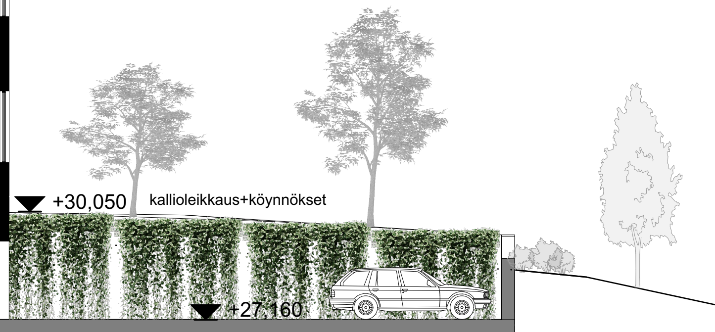
LEIKKAUS A-A
