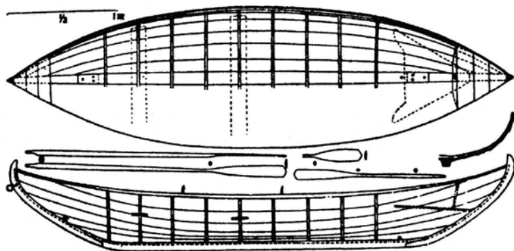
63. Laatokan vene.
